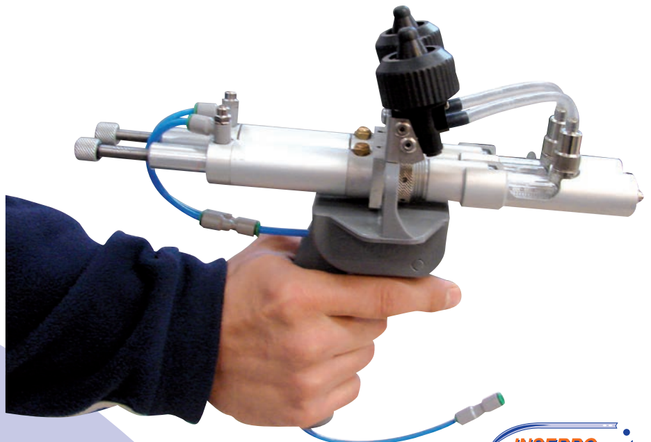
JN-140 Jeringa neumática de 2+2 ml con portafascos
