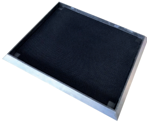
IA-677A Pediluvio de desinfección caucho 28 l, 985 x 810 x 50 mm,
