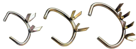
Destetador metálico para tenaza Metallic milk sucking preventor
