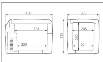
Dimensiones 14L
