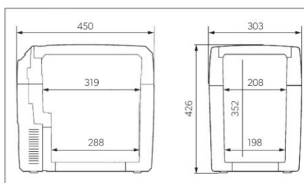
Dimensiones 21L
