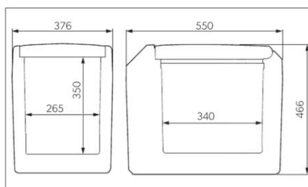
Dimensiones 35L
